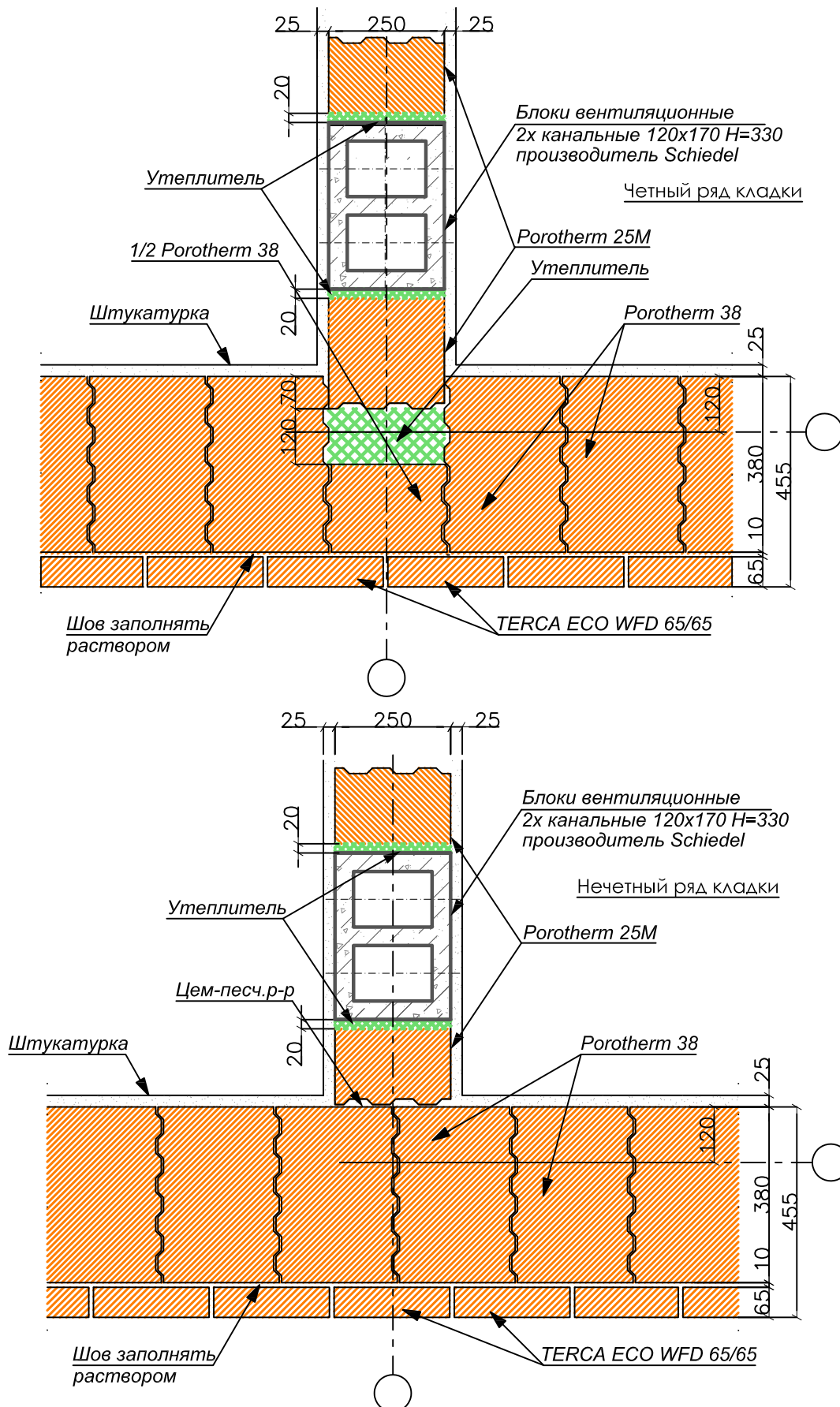
Узел сопряжения наружной стены тип 2 из Porotherm 38 с внутренней стеной из Porotherm 25М
